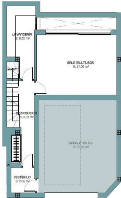
PLANTA SÓTANO
